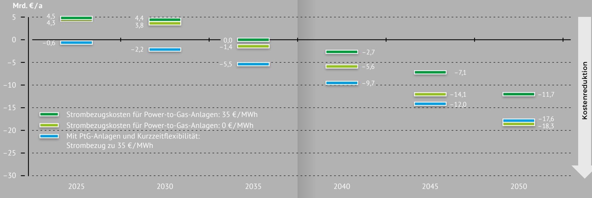
Abbildung: Kosteneinsparung der Stromversorgung mit Power-to-Gas-Anlagen für den Ausgleich der fluktuierenden Einspeisung Erneuerbarer Energien im Vergleich zu einem Stromversorgungssystem ohne Power-to-Gas, welches seine Flexibilität ausschließlich mittels Erdgas aus konventionellen Gaskraftwerken bezieht. Basierend auf den Rahmenbedingungen von Sterner et al. (2015) und Götz et al. (2016) sind folgende Szenarien dargestellt: Einsatz von Power-to-Gas-Anlagen bei Strombezugskosten zu 0 €/MWh (optimistisch-kostengünstigster Fall), zu 35 €/MWh (Abschätzung der Zahlungsbereitschaft für Base-Preis) und zu 35 €/MWh in Kombination mit Kurzzeitflexibilitätsoptionen (Batterien, Power-to-Heat).
